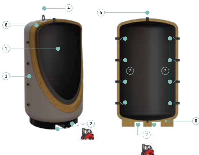
ESQUEMA DEPÓSITO
