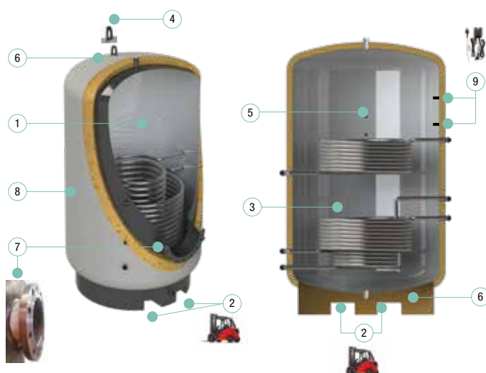
ESQUEMA DEPÓSITO
