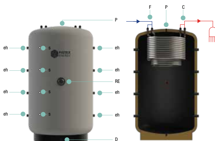
ESQUEMA CONEXIONES
