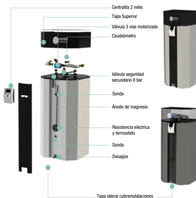
DEPÓSITO CON DESGLOSE DE ELEMENTOS
