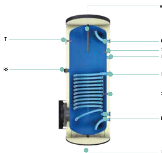
ESQUEMA CONEXIONES
