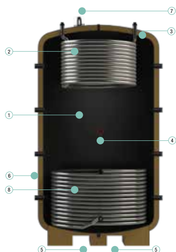
ESQUEMA DEPÓSITO
