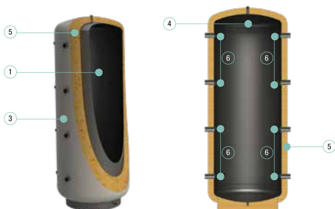
ESQUEMA DEPÓSITO
