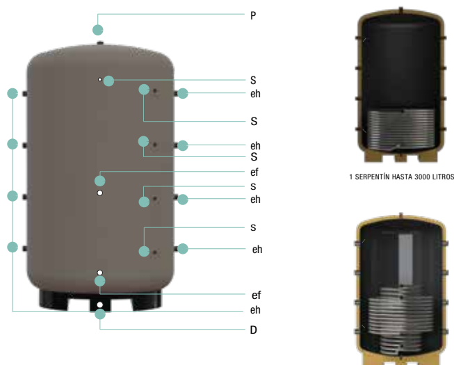
ESQUEMA CONEXIONES
