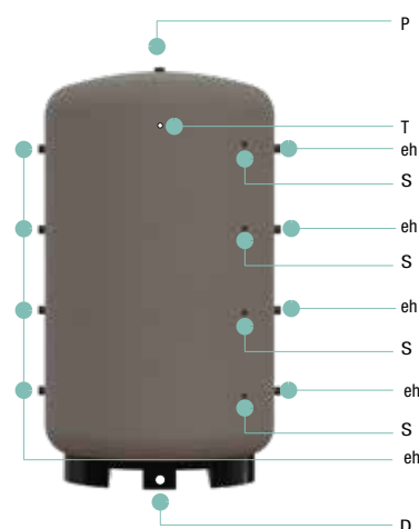
ESQUEMA CONEXIONES
