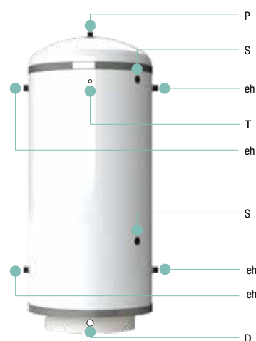
ESQUEMA CONEXIONES
