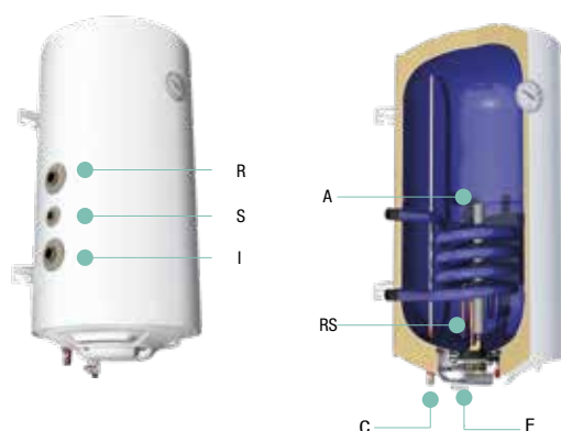
ESQUEMA CONEXIONES 80, 100 y 120
