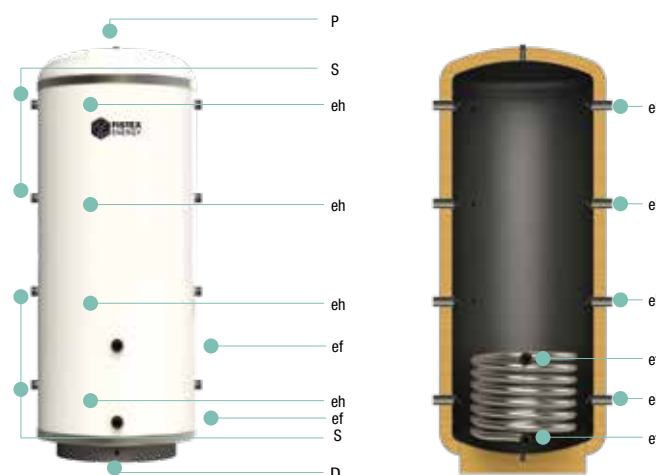
ESQUEMA CONEXIONES
