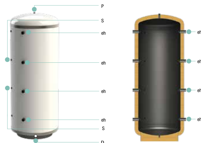
ESQUEMA CONEXIONES
