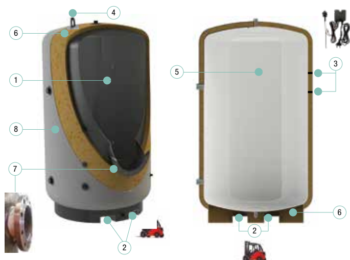
ESQUEMA DEPÓSITO
