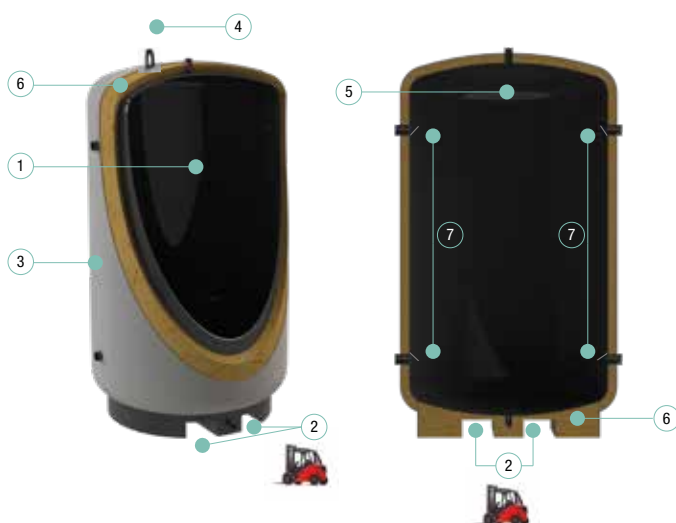
ESQUEMA DEPÓSITO
