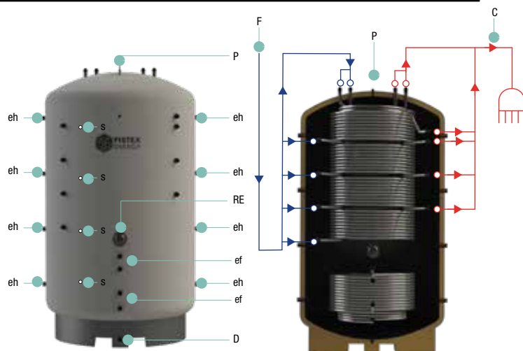
ESQUEMA CONEXIONES
