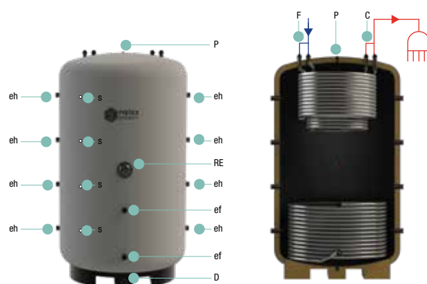
ESQUEMA CONEXIONES
