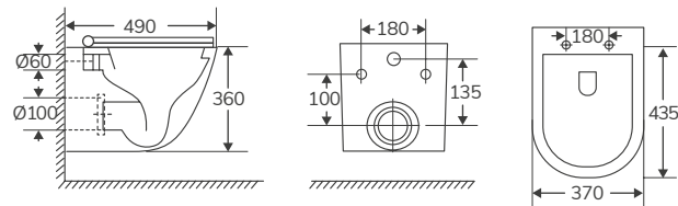
GÉNOVA SUSPENDIDO PARA CISTERNA EMPOTRADA (incluye tapa)
