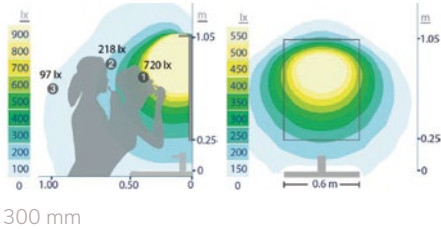
CURVAS FOTOMÉTRICAS
