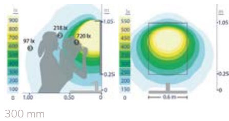
CURVAS FOTOMÉTRICAS
