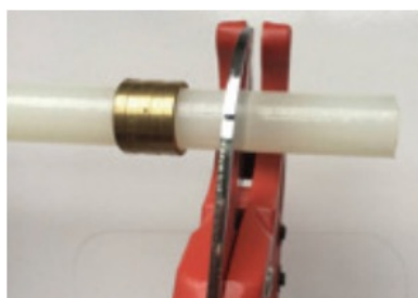
1. Cortar el tubo en ángulo recto. 1. Cortar o tubo em ângulo recto.
