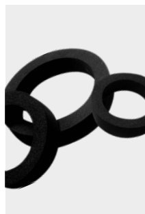
Kit Juntas KJ 2 Ref. 0138548020 Granel 50 uds/caja PVP: 1,88 € Ø 111 / 82 / 56 mm x 15 Espesor
