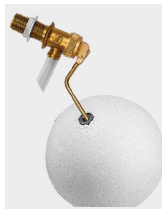
GPB 2 Ref. 0151551530 Packaging Bolsa 25 uds/caja PVP: 9,67 € Grifo lateral (Latón) + Tuerca (Plástico) + Boya Ø 3/8" Latón + Longitud: 32 mm
