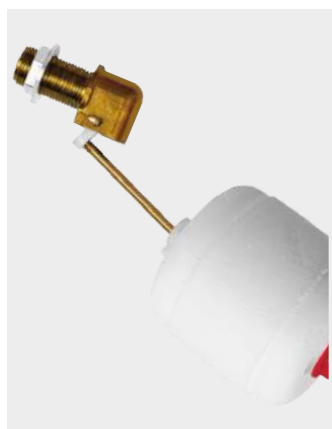
GCB 1 Ref. 0151650630 Packaging Bolsa 25 uds/caja PVP: 6,04 € Grifo lateral (Latón) + Tuerca + Boya Ø 3/8" Latón + Longitud: 30 mm
