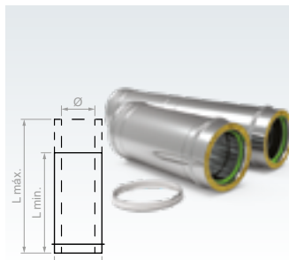
TUBO TELESCÓPICO DE 500 A 900 MM. MACHO - HEMBRA (ACERO INOXIDABLE)
