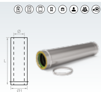
TUBO DE LONGITUD 1000 MM. MACHO - HEMBRA (ACERO INOXIDABLE)
