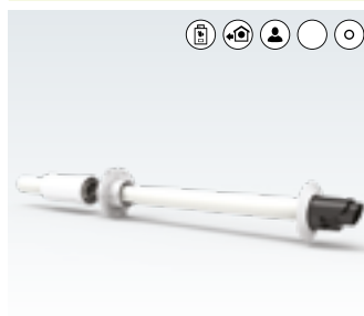
610KCCSUST55 KIT HORIZONTAL Ø60/100 COMPATIBLE PARA CALDERAS
