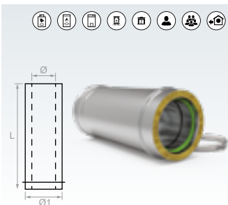
TUBO DE LONGITUD 500 MM. MACHO - HEMBRA (ACERO INOXIDABLE)
