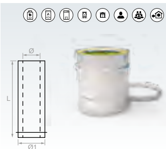
TUBO DE LONGITUD 250 MM. MACHO - HEMBRA (ACERO INOXIDABLE)
